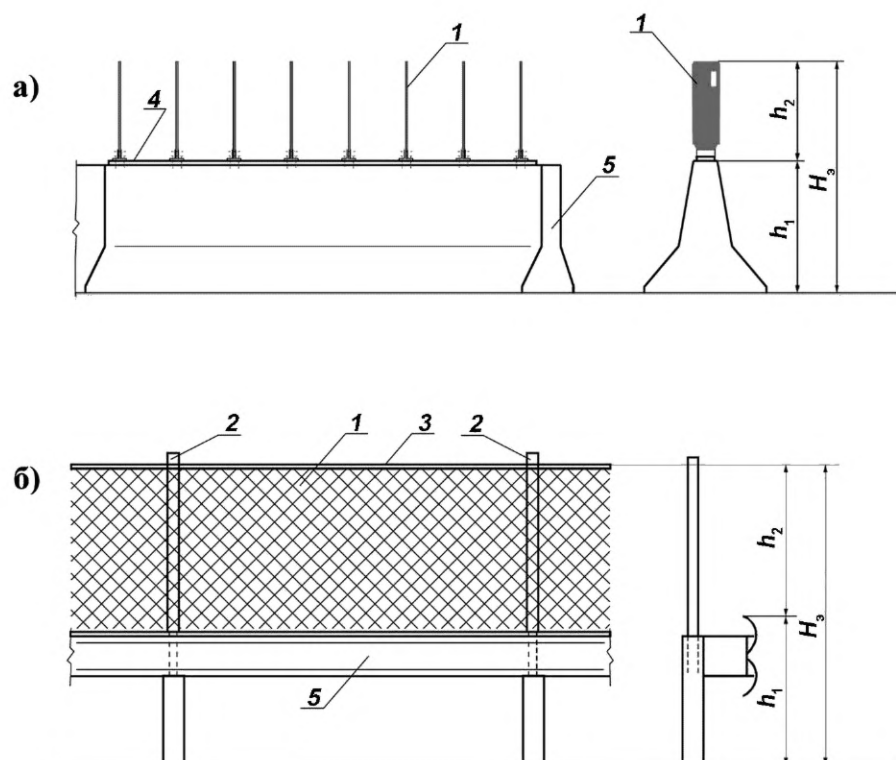
1 — затеняющий элемент; 2 — стойки; 3 — рейки; 4 — опора; 5 — основание (ограждение барьерного или парапетного типа); h_1 — высота ограждения; h_2 — высота затеняющего элемента; H_3 — эффективная высота экрана
