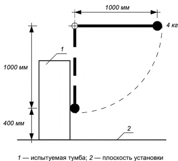
Рисунок 4 — Испытание на малую динамическую нагрузку
