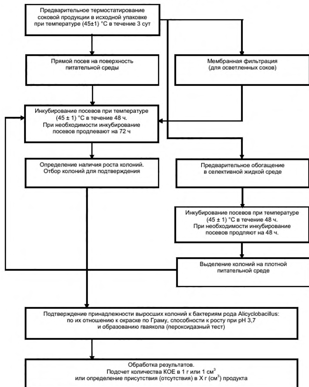
Рисунок Г.1 - Схема выявления и определения количества бактерий рода Alicyclobacillus в готовой соковой продукции
