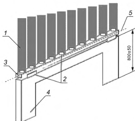
1 — затеняющий элемент; 2 — элемент крепления; 3 — опора; 4 — пример основы; 5 — главная ось системы
