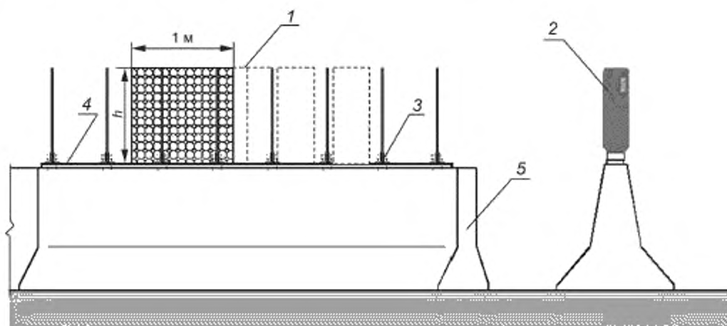
Рисунок 1 — Пример вычисления боковой видимости противоослепляющего экрана
