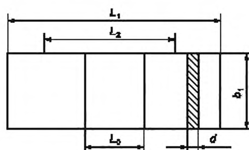
Рисунок В.1 — Образец 3-го типа
