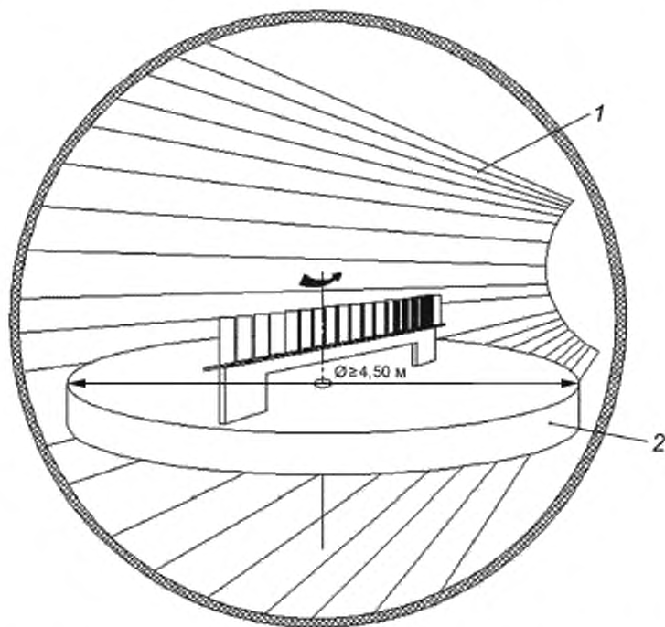
1 — рабочая секция; 2 — поворотный стол, позволяющий вращаться образцу от -90^\circ до +90^\circ
