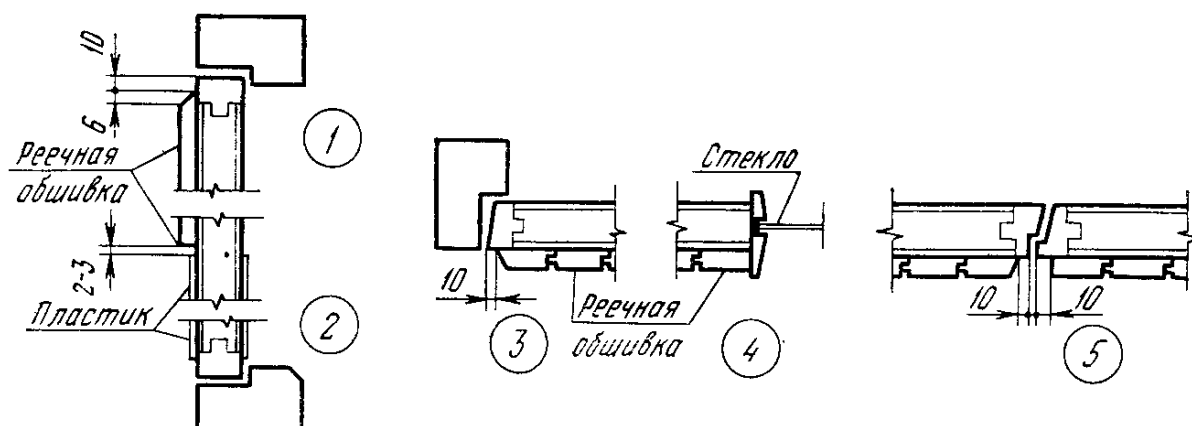
Профили реек
