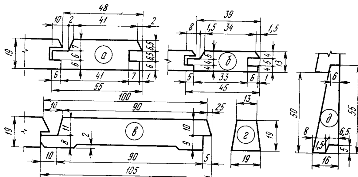
Профили реек
