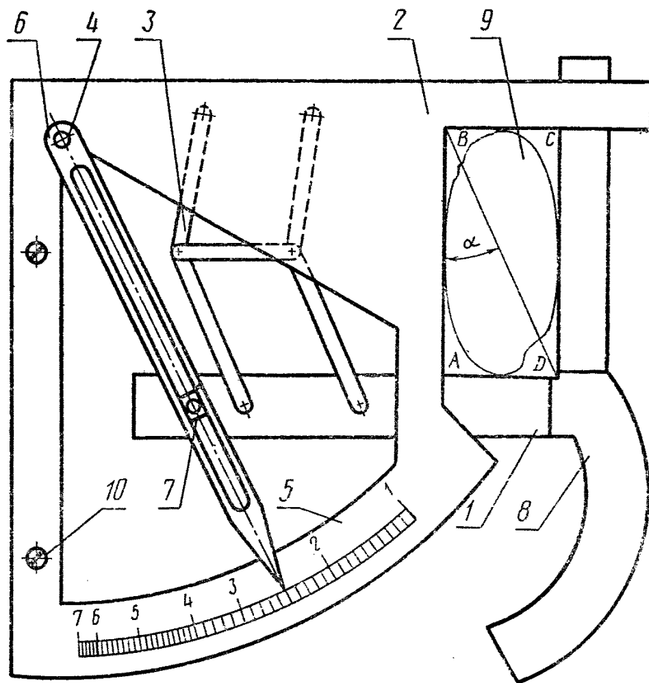
1 — подвижный угольник; 2 — неподвижный угольник; 3 — двойной шарнирный параллелограмм; 4 — кулиса-стрелка; 5 — шкала; 6 — ось поворота; 7 — ось ползуна; 8 — рукоятка; 9 — зерно щебня
