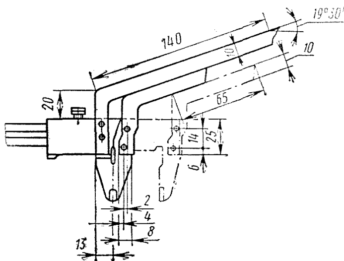
Передвижной шаблон
