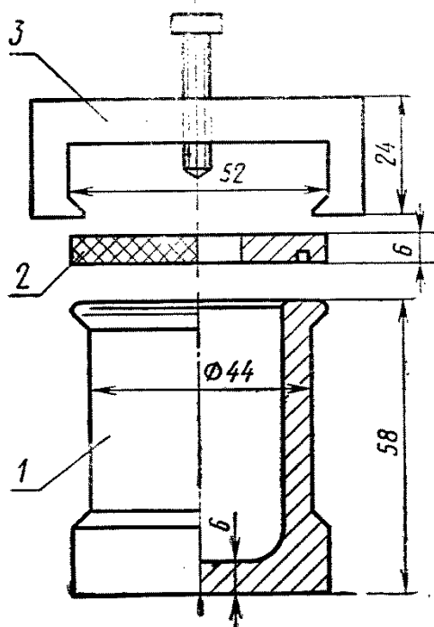
1 — корпус; 2 — крышка; 3 — захват Черт. 1
