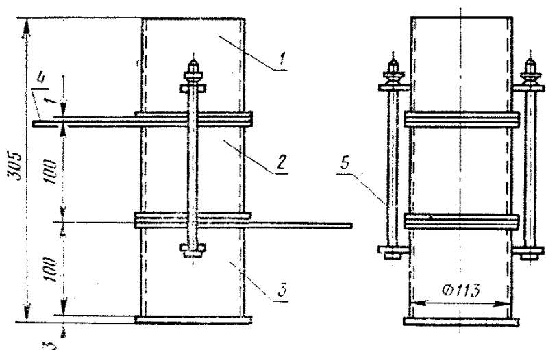
1, 2 — кольца; 3 — цилиндр; 4 и 5 — платформы
