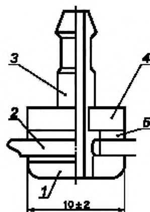
Рисунок 1 — Штуцер
