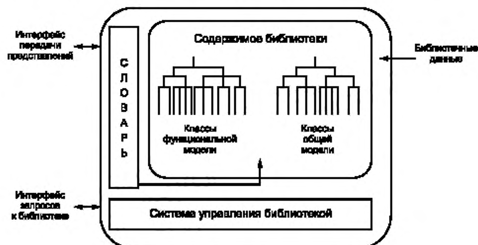
Рисунок 2 — Библиотечная система
