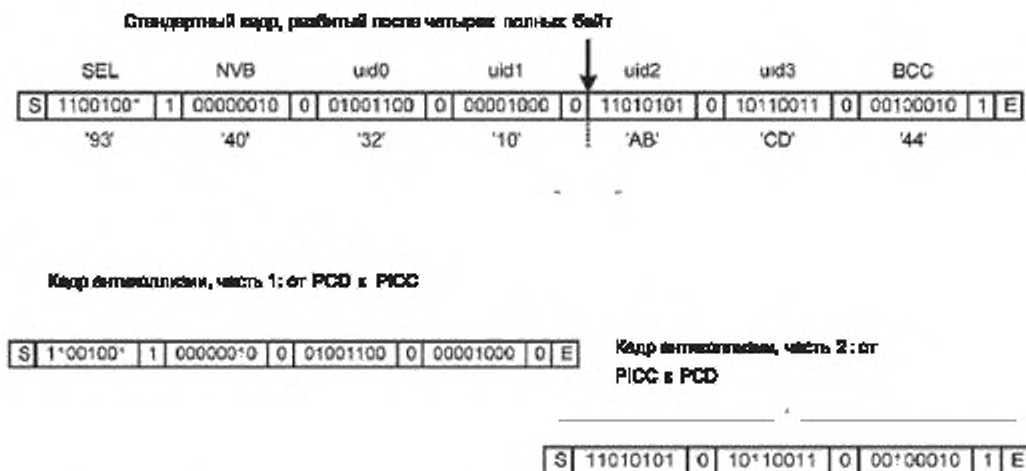
Рисунок 5 – Организация бит и передача бит-ориентированного кадра антиколлизии, случай FULL BYTE
