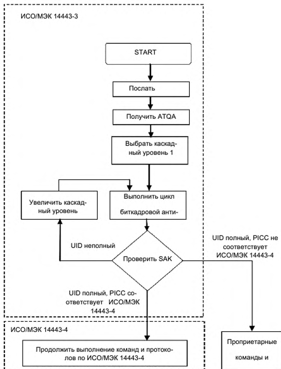
Рисунок 9 – Блок-схема инициализации и антиколлизии для PCD
