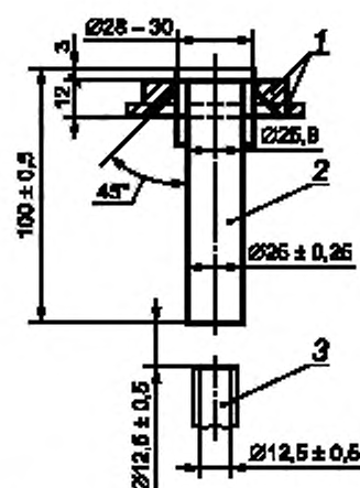
1 — держатель; 2 — образец; 3 — сопло
