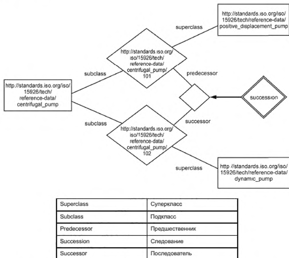
Рисунок Н.5 — Порядок «следования» как инстанцирование типов сущности по ISO 15926-2
