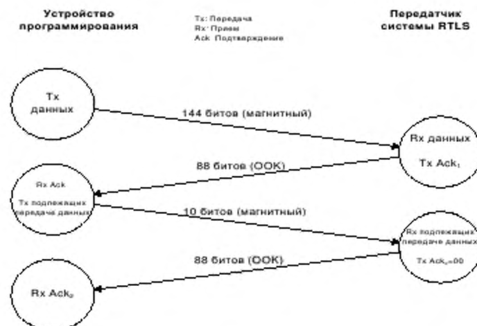
Рисунок 9 — Обмен сообщениями между устройством программирования и передатчиком системы RTLS для записи данных
