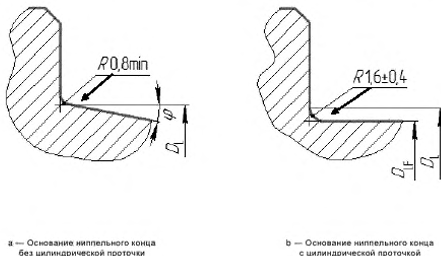
Рисунок 5 — Форма основания ниппельного конца
