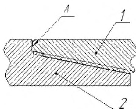
в) Расположение муфтового и nippleного концов при ручном свинчивании
