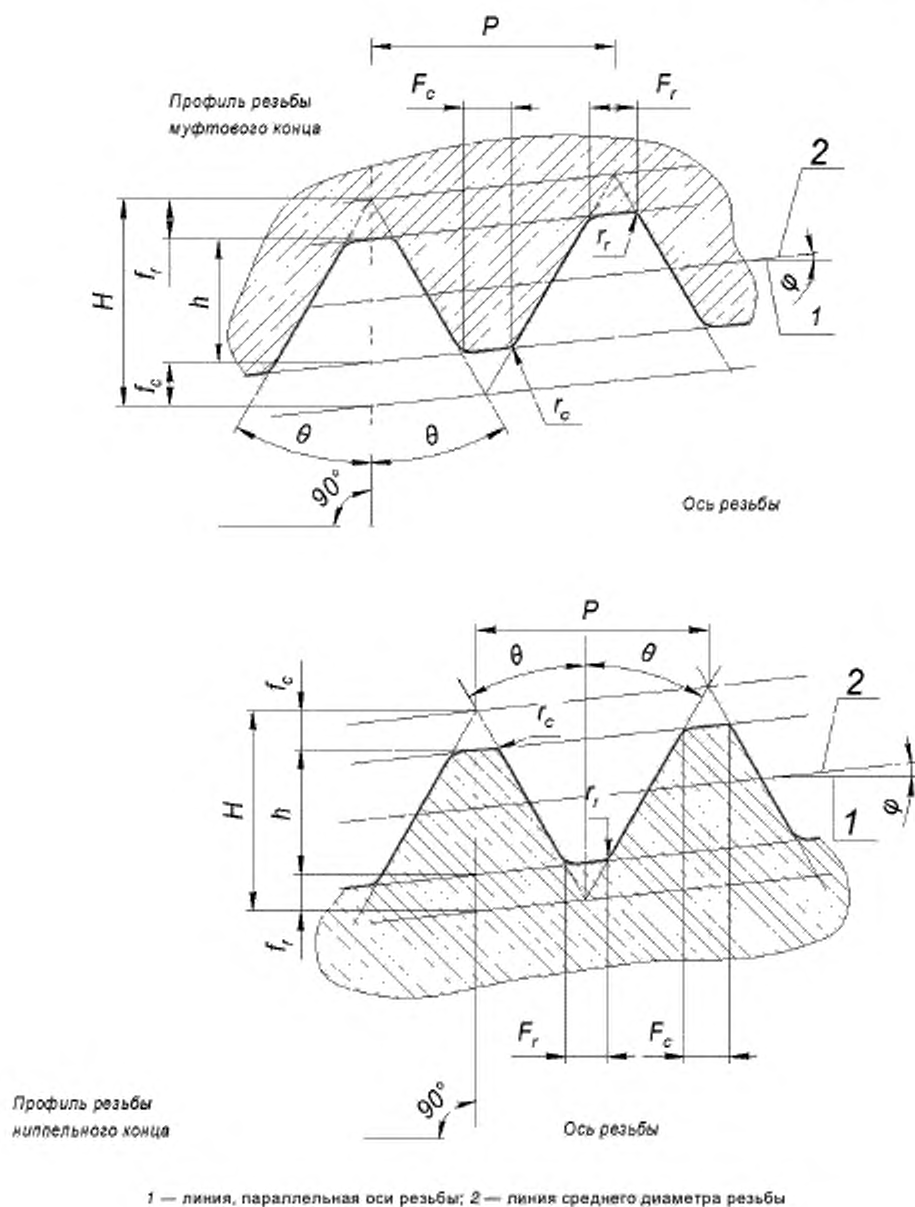
Рисунок 2 — Профиль резьбы V-055
