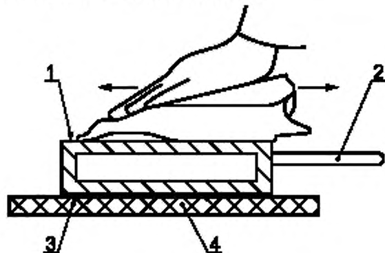
Рисунок 2 — Электризация корпуса батареи методом трения—скользящего с использованием нейлоновой ткани
