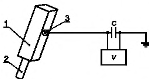
1 — корпус с накопленным зарядом; 2 — тefлоновая ручка; 3 — сферический электрод диаметром 15 мм; V — вольтметр; C — конденсатор емкостью 0,1 мкФ
