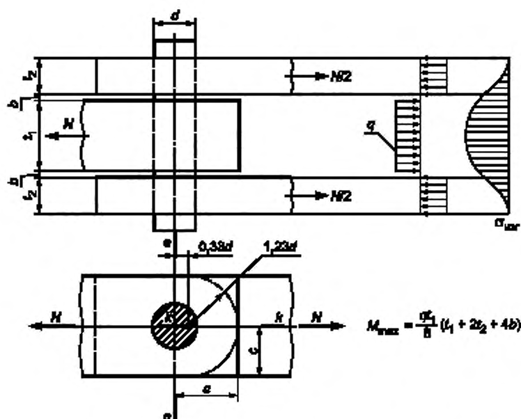
Рисунок Н.1 — Конструктивная и расчетная схема пальцевого соединения
