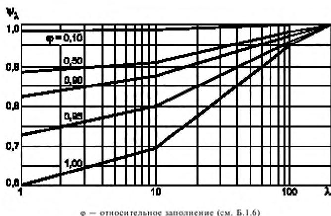
Рисунок Б.5 — Коэффициент \psi_\lambda , учитывающий относительное удлинение \lambda плоских и пространственных ферм ( \lambda = l/b ), (см. рисунок Б.4)
