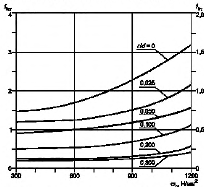
Рисунок И.2 — График для определения значений коэффициентов f_k в формуле (И.1)
