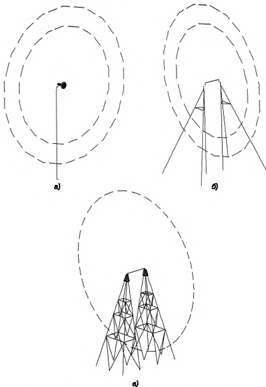
Рисунок Б.8 — Характерные конструктивные формы опор колес обозрения
