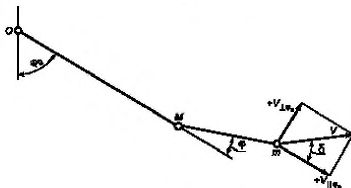
Рисунок В.5 — Разложение скорости V
