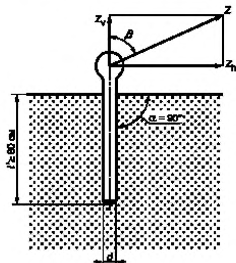
Рисунок Е.1 — Схема стержневого анкера
