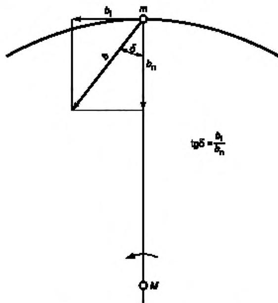
Рисунок В.6 — Направление ускорения b
