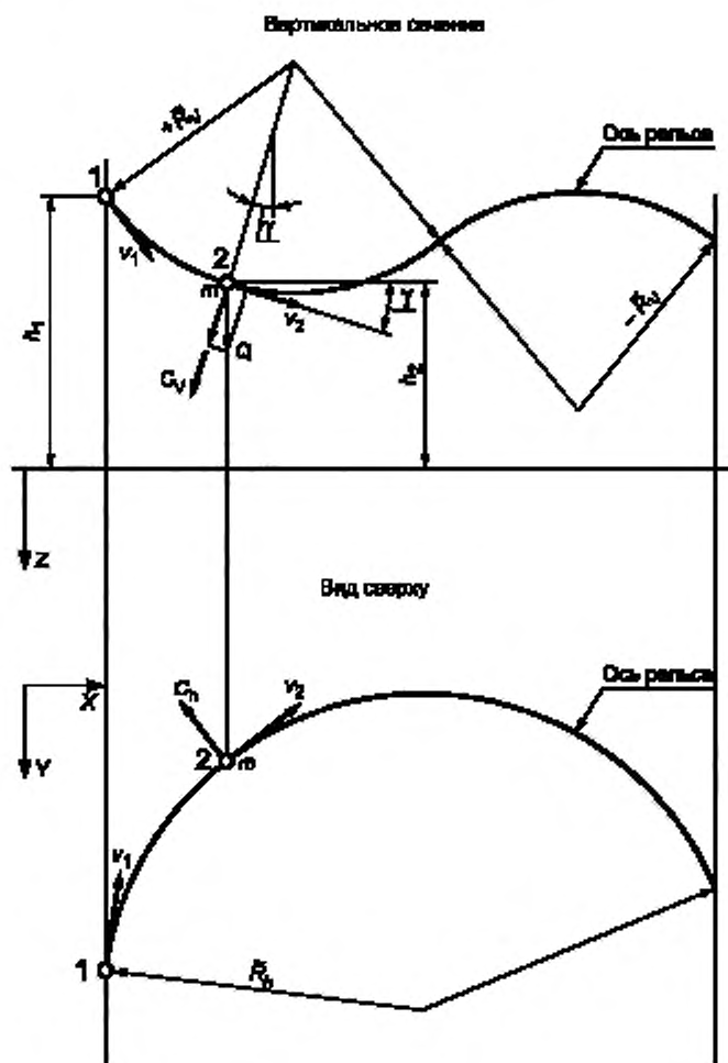
Рисунок В.7 — Вертикальное сечение и вид сверху рельсовой колес
