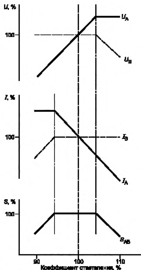
Рисунок 3 — Комбинированное регулирование напряжения (режим a )
