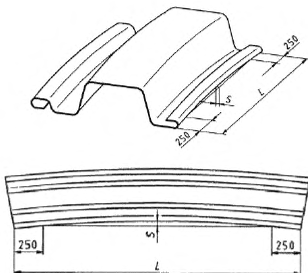
Рисунок 1 – Измерение отклонения от прямолинейности в горизонтальной плоскости
