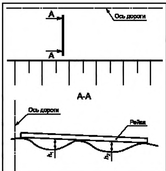
Рисунок 1 — Схема проведения измерений величины колейности
