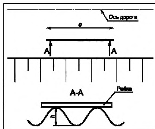
a — максимальный размер повреждения в направлении, параллельном оси автомобильной дороги, см; h — максимальный просвет под трехметровой рейкой, мм
