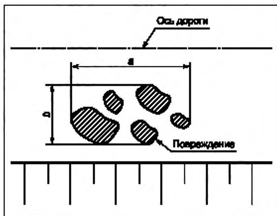
а — максимальный размер повреждения в направлении, параллельном оси автомобильной дороги, см; б — максимальный размер повреждения в направлении, перпендикулярном к оси автомобильной дороги, см
