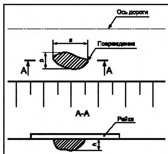
h — максимальный просвет под трехметровой рейкой, мм; a — максимальный размер повреждения в направлении, параллельном оси автомобильной дороги, см, b — максимальный размер повреждения в направлении, перпендикулярном к оси автомобильной дороги, см
