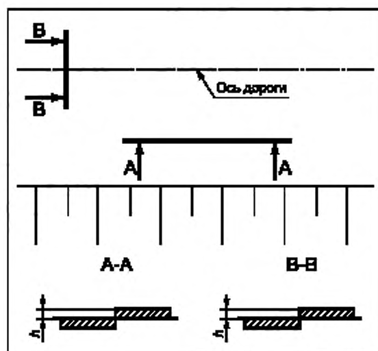
Рисунок 8 — Схема проведения измерений величины вертикального смещения дорожных плит
