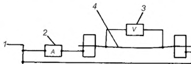
Рисунок А.4 — Электрическая схема испытания
