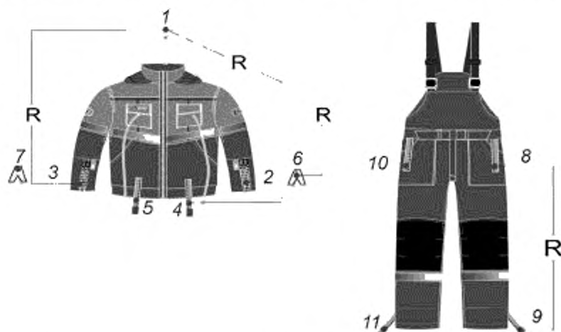
1 — верхний контактный вывод куртки; 2, 3 — контактные выводы рукавов куртки; 4, 5 — нижние контактные выводы куртки; 6, 7 — контактные зажимы переноса потенциала; 8, 10 — верхние контактные выводы полукombineзона; 9, 11 — нижние контактные выводы полукombineзона
