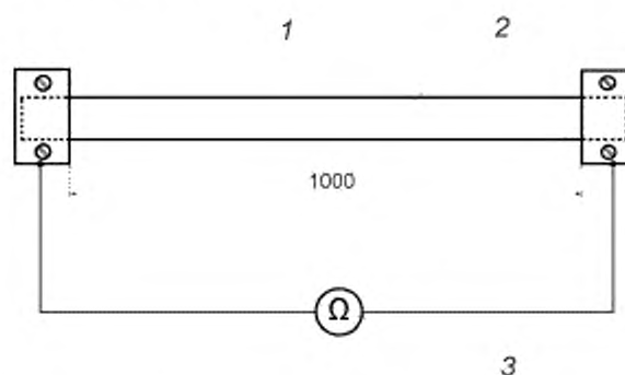
1 — разборные двоянные медные пластины; 2 — испытуемый образец; 3 — омметр
