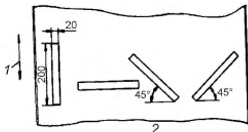
Рисунок А.3 — Пример вырезания образцов из ткани
