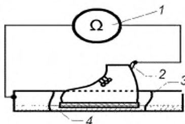
1 — омметр; 2 — контактный вывод; 3 — ванна; 4 — раствор поваренной соли
