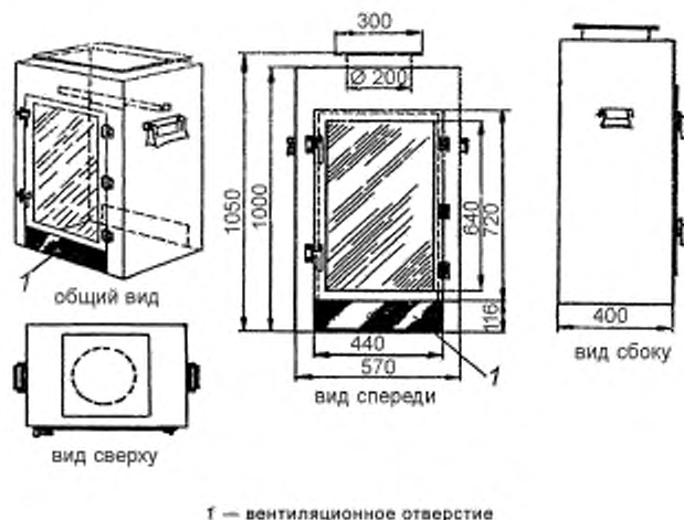
Рисунок Б.1 — Испытательная камера
