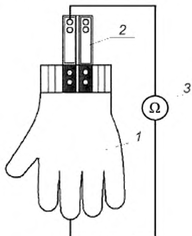
1 — защитная перчатка; 2 — контактный вывод; 3 — омметр
