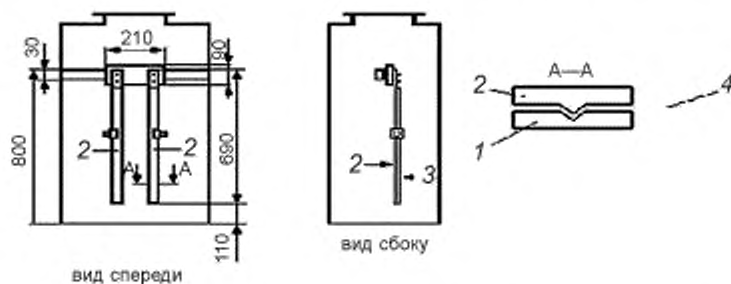
1 — неподвижная поддерживающая конструкция; 2 — съемная полоса; 3 — прижимающая полоса; 4 — испытуемый образец
