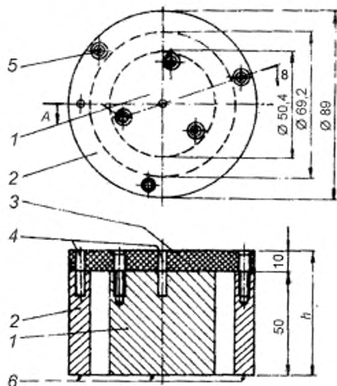
1 — внутренний цилиндрический электрод; 2 — внешний кольцевой электрод; 3 — изолирующий пластмассовый диск; 4 — отверстия для присоединения токопроводящих проводников; 5 — винты, скрепляющие конструкцию; б — поверхность системы электродов, находящаяся в контакте с образцом
