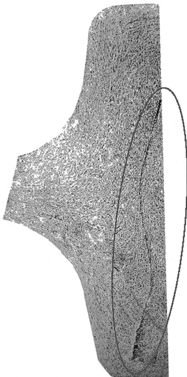
Рисунок Б.33 – Эталон № 33 (ликвационные полосы, выходящие на поверхность ступицы)
