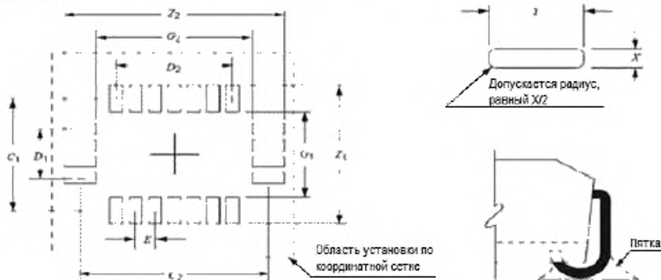
Рисунок 8 – Размеры посадочного места прямоугольного компонента QFJ, лист 1
