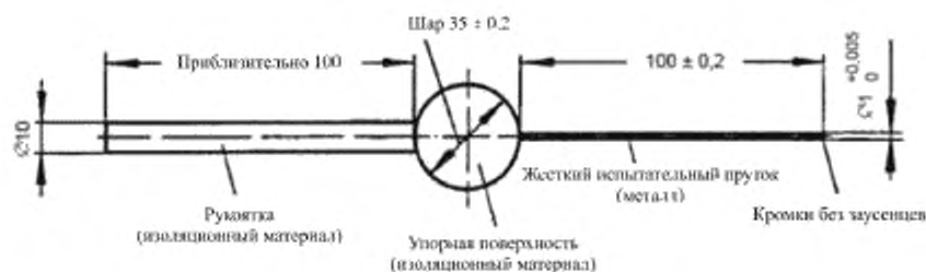
Рисунок V.5 — Щуп для испытания клемм
