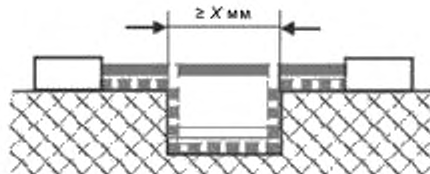
Рисунок О.1 — Узкая канавка
