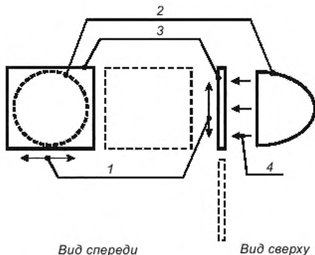
1 — направление движения экрана; 2 — устройство освещения; 3 — экран; 4 — направление светового потока
