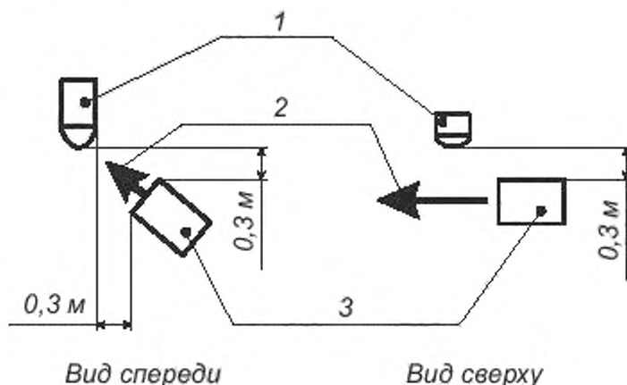
1 — ПОЭИ; 2 — направление потока воздуха; 3 — тепловентилятор
