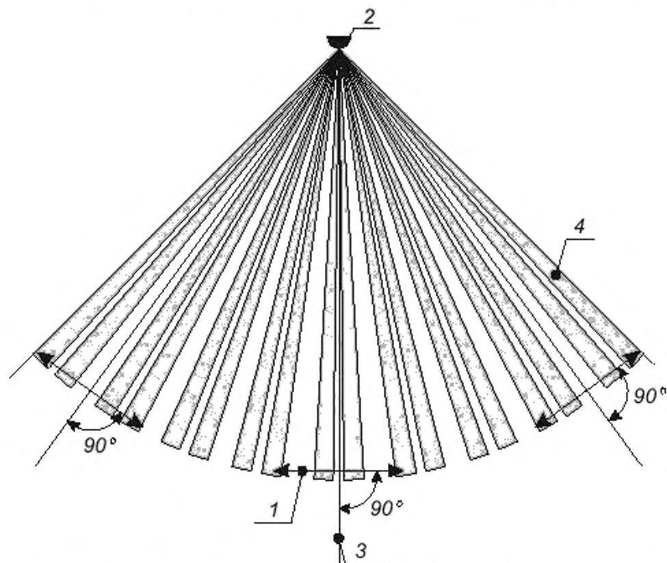
Рисунок А.1 — Испытание по 5.4.1 (таблица 3, позиции 1 и 3) и 5.5.1 (таблица 10, позиции 1 и 3)
