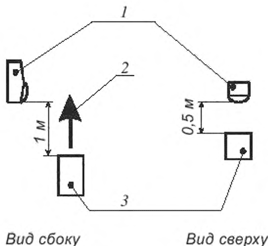
1 — ПОЭИ; 2 — направление потока воздуха; 3 — тепловентилятор
