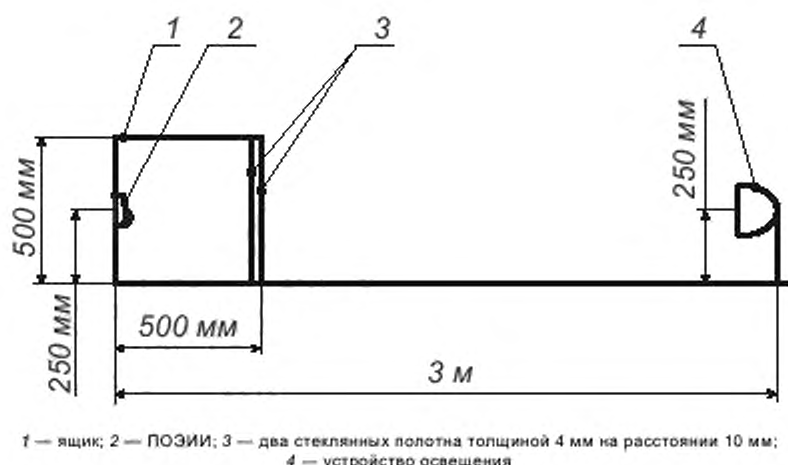
Рисунок 4 — Схема проведения испытаний на устойчивость к внешней засветке
