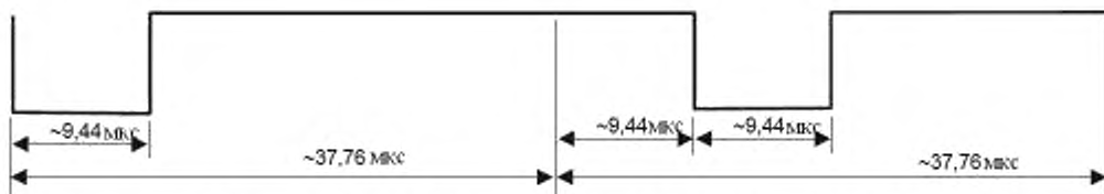
Рисунок 8 – Начало кадра при способе кодирования «1 из 4»
