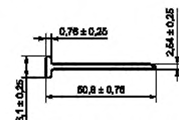
Рисунок 2а — размеры испытательного снаряда из гвоздя
