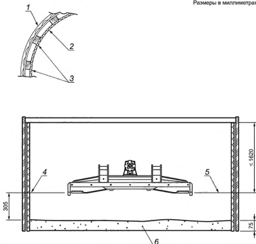
1 — вторичная стена; 2 — стены-мишени; 3 — подложки стен-мишеней; 4 — линия расположения режущих элементов; 5 — горизонтальная плоскость расположения неподвижных режущих элементов
