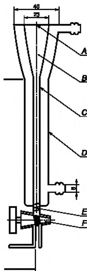
A — место соединения с муфтой из матового стекла. B — свободное пространство; C — внутренняя часть колонки. D — внешняя часть колонки; E — пробка из стекловолны; F — запорный кран
