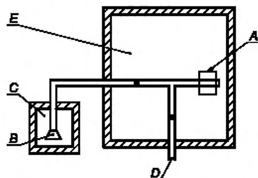
А — сенсорная головка вращающегося ротора, В — ячейка с образцом, С — термостат; D — соединение с вакуумом (турбо насос); E — воздушный термостат
