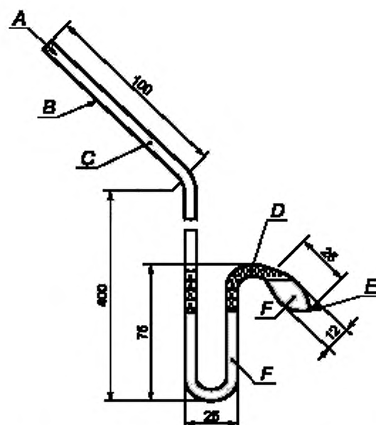
А — устройство регулирования давления; В — трубка (наружным диаметром 8 мм); С — осушенный азот в системе давления; D — пар образца; E — маленький наконечник; F — жидкий образец
