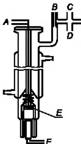
А — термодпара; В — вакуумный буферный объем; С — датчик давления; D — соединение с вакуумом; E — точка измерения; F — электронагревательный элемент с.а. 150 Вт
