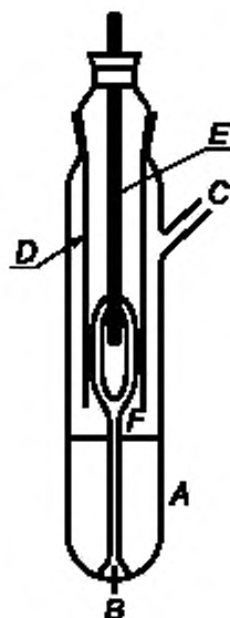
А — трубка, содержащая кипящую жидкость; В — платиновый провод, вмонтированный в дно; С — боковая трубка; D — кожух, Е — термометр; F — плечо насоса
