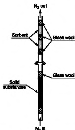
Рисунок 9 — Стекло́нная трубка для твердых образцов
