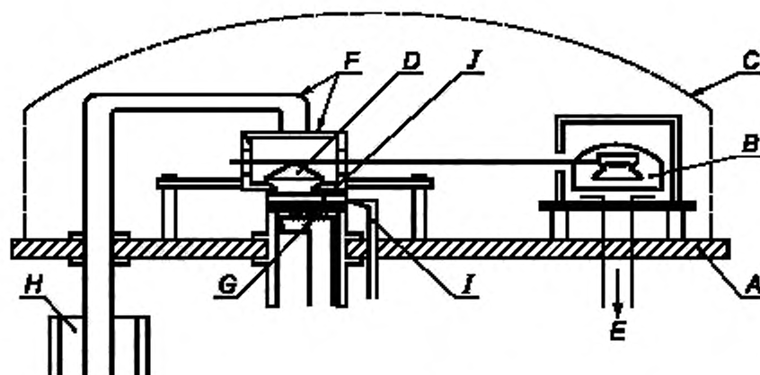
А — основание; В — вращающаяся катушка; С — вакуумный колпак; D — весы с чашками; E — устройство измерения вакуума; F — холодильная камера; G — печь — испаритель; H — сосуд Дьюара с жидким азотом; I — измерение температуры образца; J — тест-вещество
