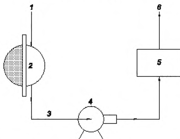
1 — подача свежей среды-носителя; 2 — камера с изнаночной стороны элементарной пробы для взятия пробы среды-носителя; 3 — взятие пробы среды-носителя; 4 — насос; 5 — анализатор проб среды-носителя; 6 — отходы испытания
