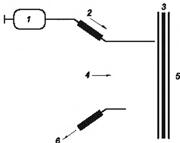
1 — шприц для ввода испытательной жидкости; 2 — введение испытательной жидкости; 3 — алюминиевая фольга или другой инертный материал; 4 — введение среды-носителя; 5 — лицевая сторона модифицированной элементарной пробы; 6 — среда-носитель на анализ.
