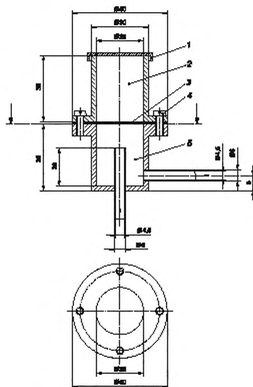
1 — открывающаяся крышка; 2 — камера для жидкости; 3 — элементарная проба материала; 4 — винты; 5 — проточная камера
