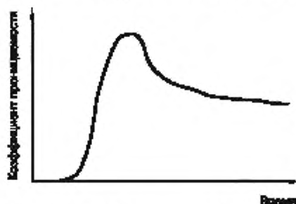
д) Тип кривой проникания, характерный для случаев, когда элементарная проба набухает, но процесс проникания стабилизируется
