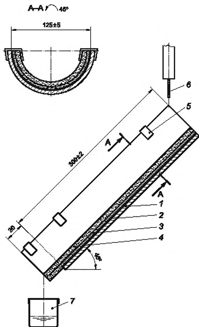
1 — желоб, 2 — прозрачная пленка; 3 — фильтровальная бумага; 4 — испытываемая элементарная проба; 5 — зажимы; 6 — игла; 7 — лабораторный стакан
