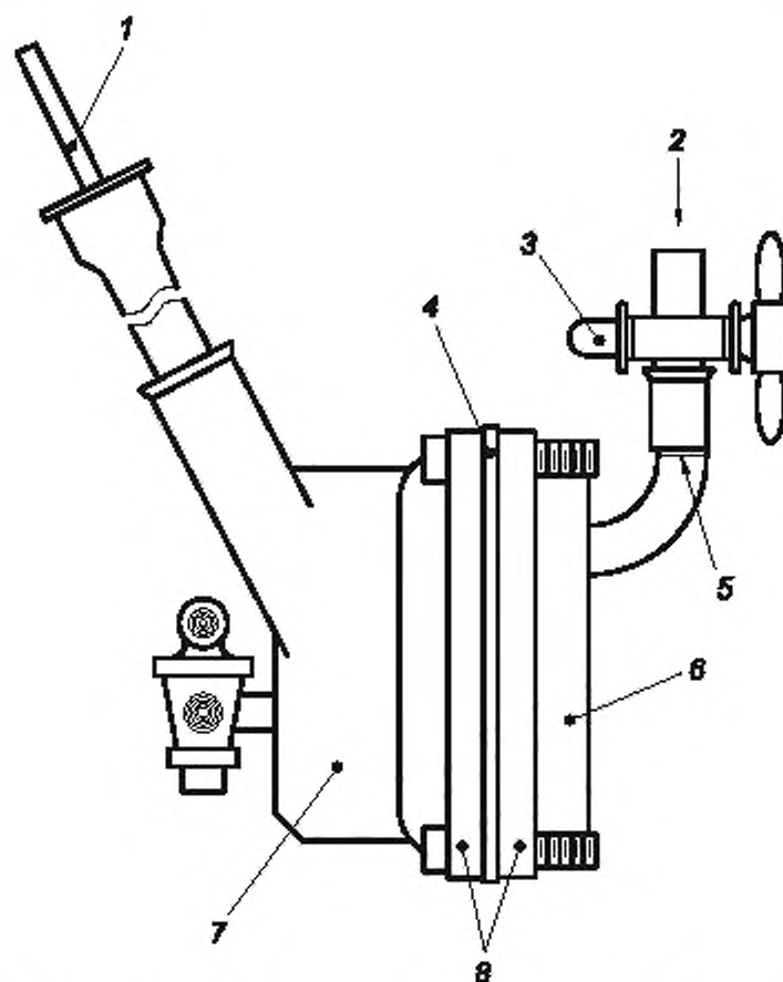
1 — сменная мешалка; 2 — впускной шланг испытательной жидкости; 3 — запорный кран; 4 — прокладка; 5 — уровень заполнения; 6 — камера с лицевой стороны образца для испытательной жидкости; 7 — камера с изнаночной стороны элементарной пробы для взятия пробы среды-носителя; 8 — алюминиевые фланцы
