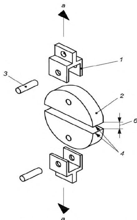
1 – вилчатый захват; 2 – поверхность полудиска, на которую устанавливают образец; 3 – фиксирующий штифт; 4 – закругленные кромки полудисков; а – направление приложения нагрузки; б – расхождение полудисков
