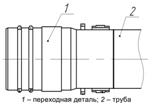
Рисунок А.4 – Переходная стальная деталь со сварным соединением
