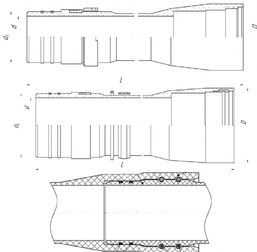
Рисунок А.5 – Варианты раструб-нипельного соединения труб
