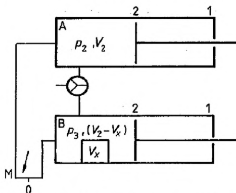
А – камера А; В – камера В; М – манометр; p_2 – давление в камере А; p_3 – давление в камере В; V_2 – объем камеры; V_x – объем образца; 0 – равновесная позиция; 1 – позиция поршня 1; 2 – позиция поршня 2
