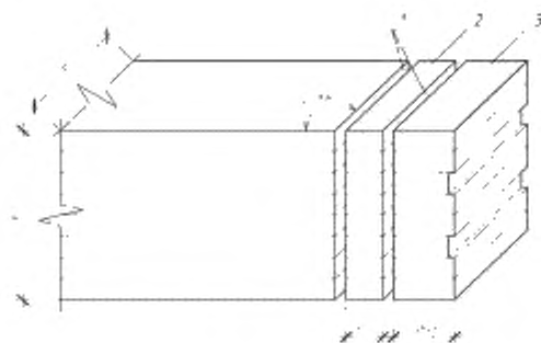
A — проектный размер конструкции; H — высота конструкции; B — ширина конструкции; 1 — пропилы; 2 — заготовка для образцов; 3 — отпад
