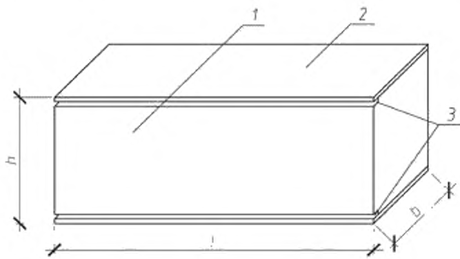
1 — древесина; 2 — древесноплитный материал; 3 — свесы
