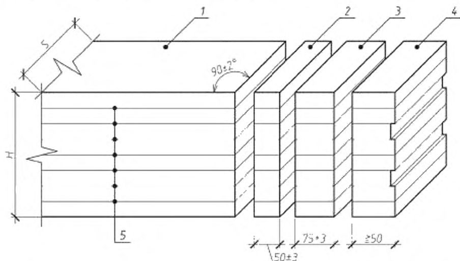
H и S — высота и ширина клеевого элемента; 1 — многослойный элемент, 2 — заготовка для выпиливания образцов для предварительных испытаний на послойное скалывание; 3 — образец для испытаний на расслаивание; 4 — торцевой срез; 5 — клеевые швы
