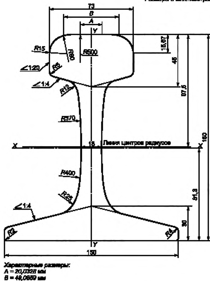
Рисунок А.3 — Рельс типа РП65
