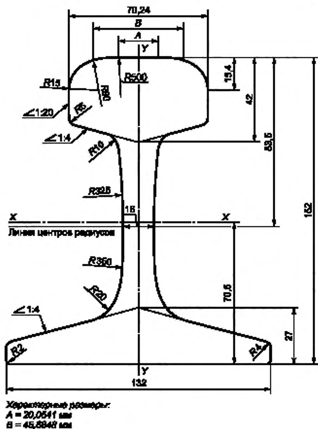
Рисунок А.1 — Рельс типа РГ50
