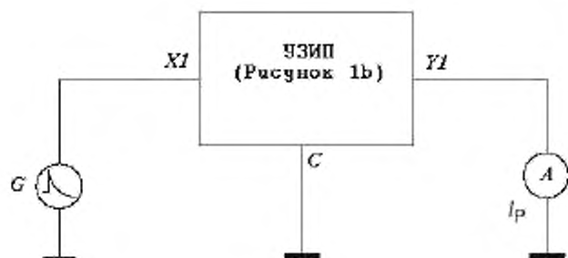
Рисунок E.2 – Определение сквозного тока общего вида
