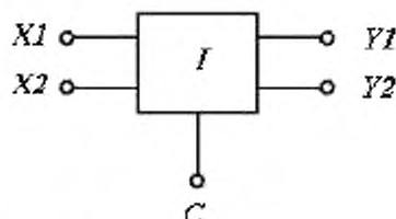
А.1д – Пятивыводной токоограничитель
