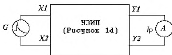
Рисунок E.3 – Определение сквозного тока дифференциального вида
