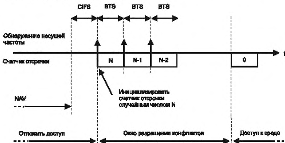
Рисунок 27 – Процедура отсрочки передачи с CSMA/CA
