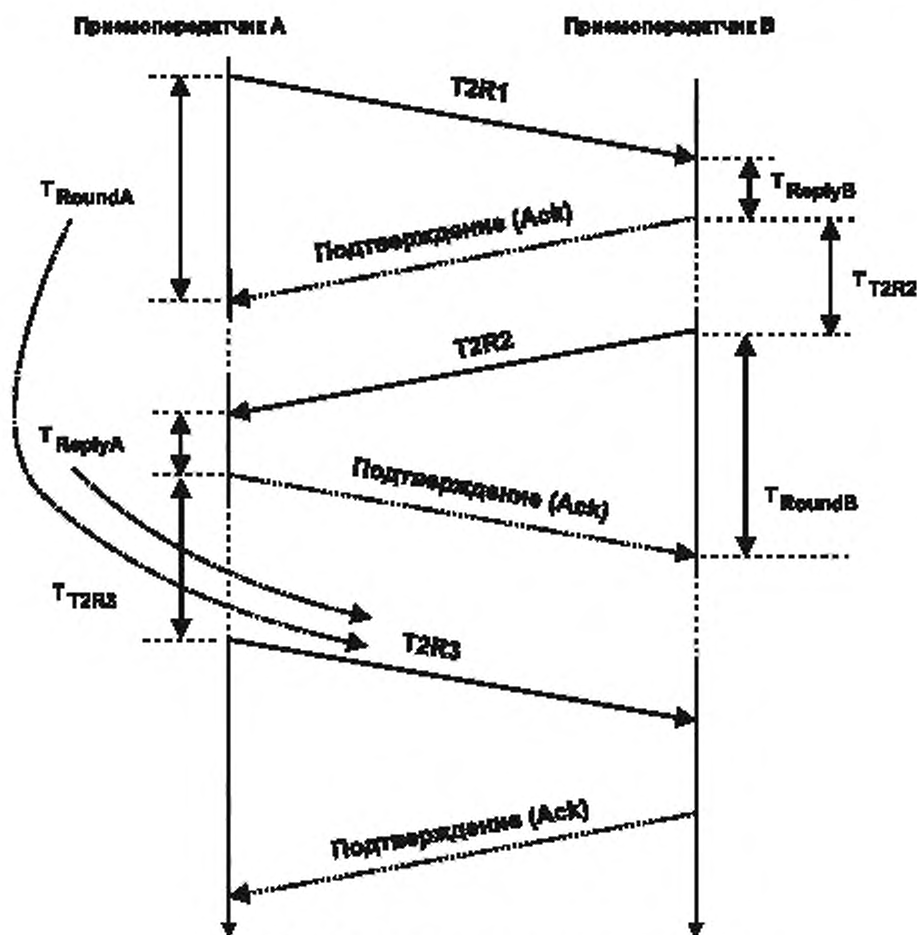
Рисунок 57 – Обмен пакетами измерения расстояния типа 2
