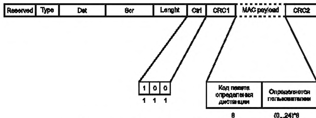
Рисунок 46 – Формат пакета измерения расстояния T1R1
