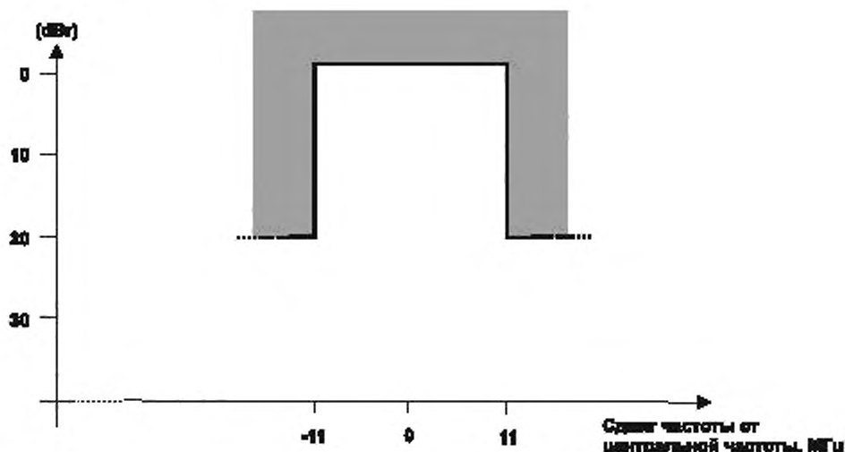
Рисунок 6 – Пределы передаваемой СПМ для двухточечной ортогональной ЛЧМ с полосой частот 22 МГц
