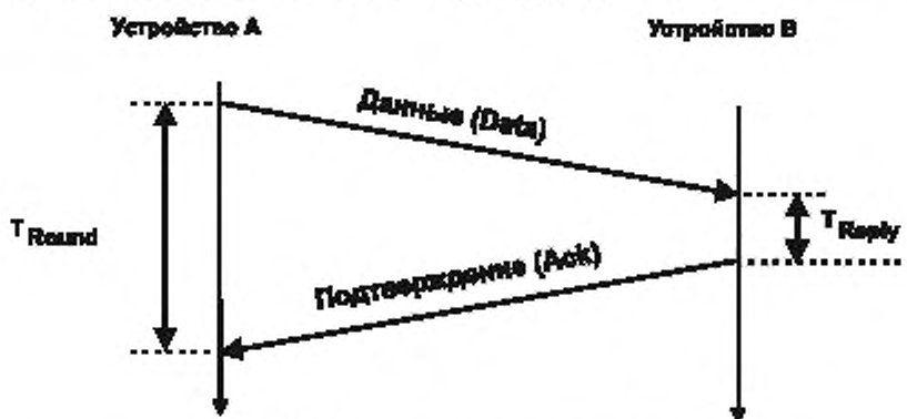
Рисунок А.1 – Двунаправленное измерение расстояния
