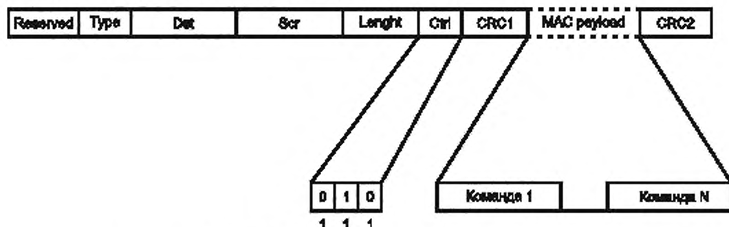
Рисунок 41 – Формат прикладного пакета команд
