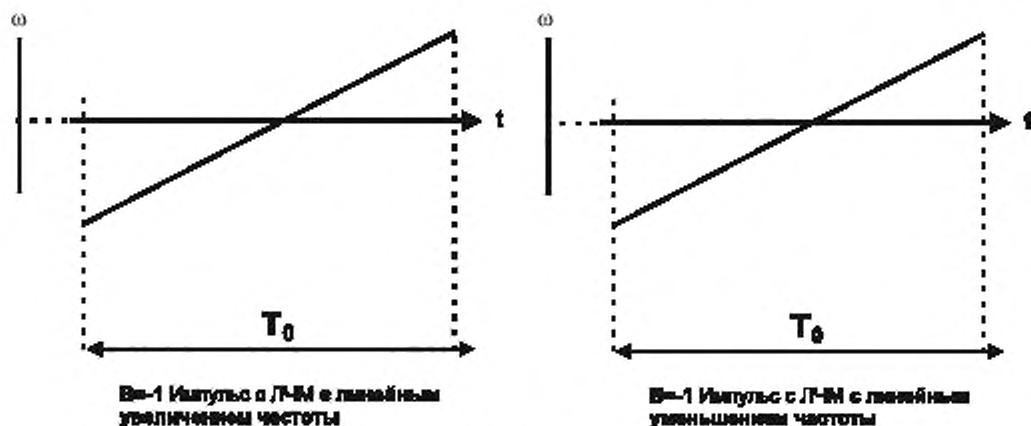
Рисунок 9 – Импульсы с ЛЧМ в частотно-временной области
