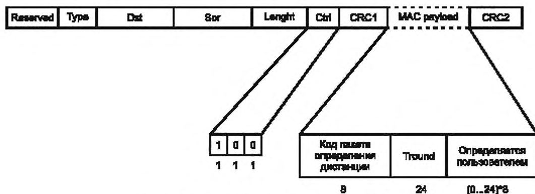
Рисунок 48 – Формат пакета измерения расстояния T1R3
