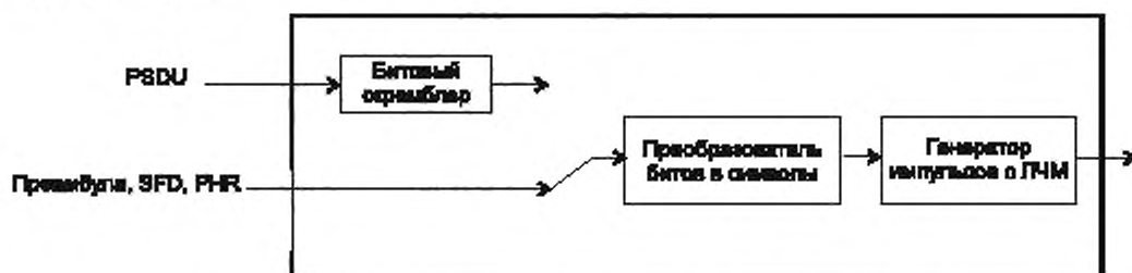
Рисунок 4 – Эталонный модулятор для двухточечной ортогональной ЛЧМ
