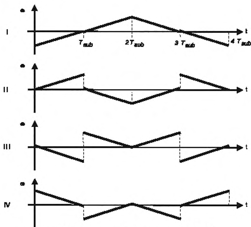
Рисунок 14 – Четыре последовательности подсигналов с ЛЧМ
