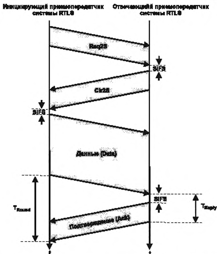
Рисунок 23 – Временные параметры пакетов «Запрос передачи» (RTS) и «Готов к приему» (CTS)
