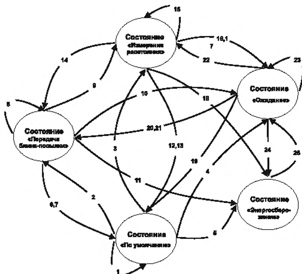
Рисунок 28 – Состояния метки на прикладном уровне
