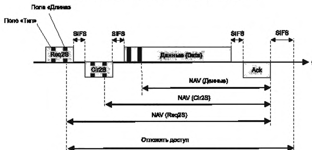
Рисунок 26 – NAV для трехэтапного установления связи
