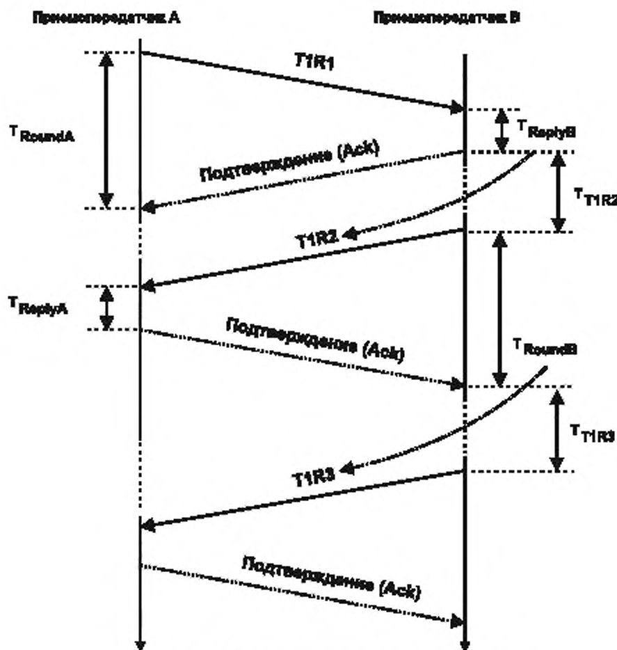
Рисунок 56 – Обмен пакетами измерения расстояния типа 1
