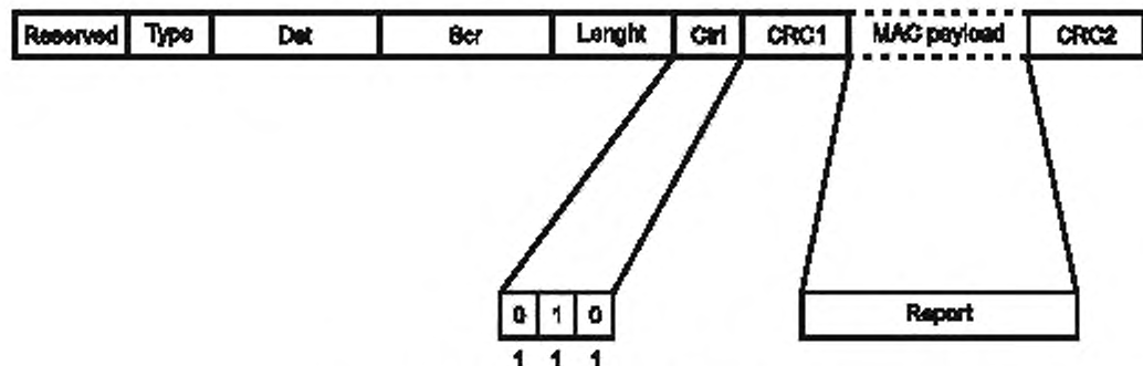
Рисунок 42 – Формат прикладных пакетов отчетов
