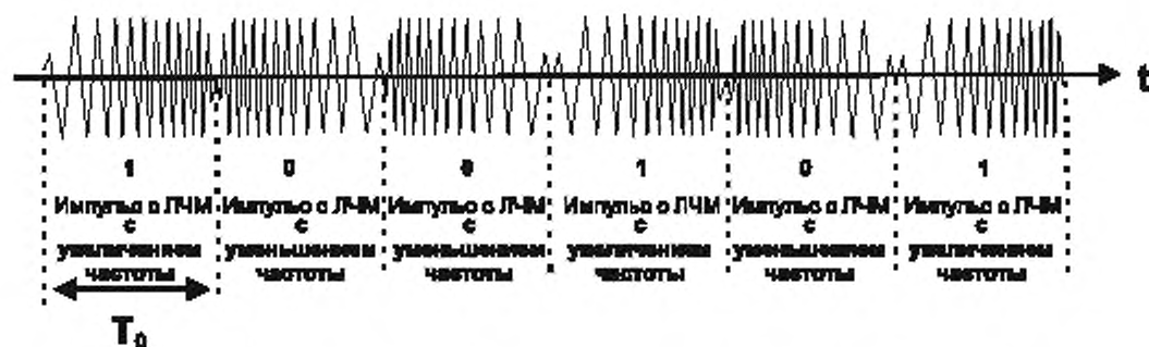
Рисунок 10 – Модулированная двоичная последовательность двухточечной ортогональной ЛЧМ
