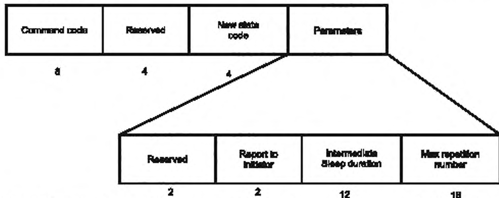
Рисунок 34 – Формат команды «Переключение в состояние «Измерение расстояния» (SwitchState(Range))
