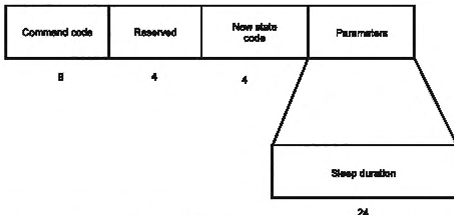
Рисунок 35 – Формат команды «Переключение в состояние «Энергосбережение» (SwitchState(Sleep))
