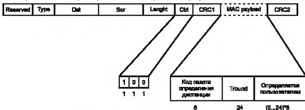
Рисунок 55 – Формат пакета измерения расстояния T4R2
