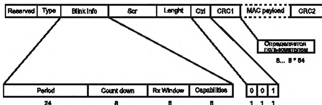
Рисунок 40 – Формат прикладного пакета передачи блинк-посылки
