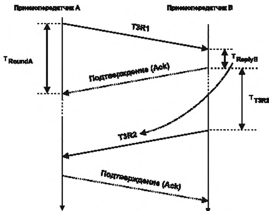
Рисунок 58 – Обмен пакетами измерения расстояния типа 3
