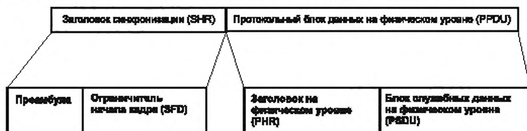
Рисунок 3 – Общая формат пакета физического уровня
