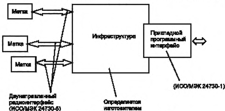
Рисунок 1 – Составные части системы RTLS
