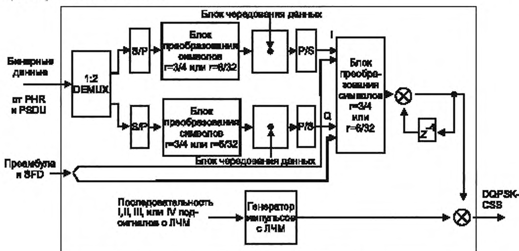
Рисунок 12 – Эталонный модулятор для DQPSK-CSS
