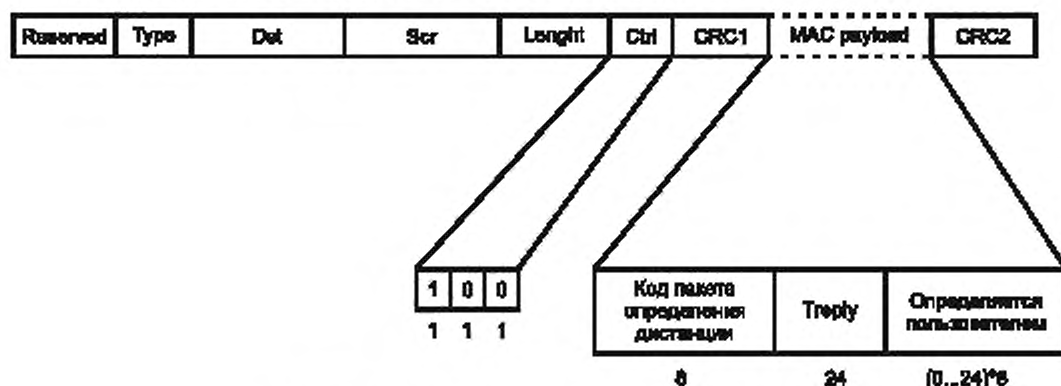
Рисунок 47 – Формат пакета измерения расстояния T1R2
