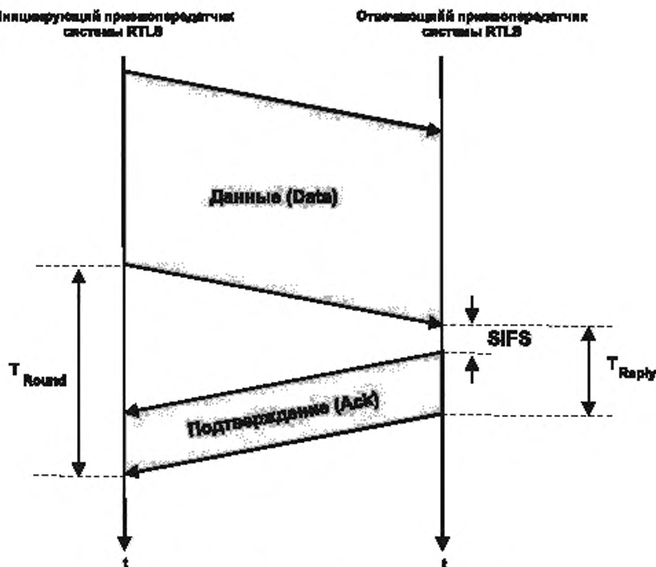
Рисунок 22 – Временные параметры подтверждения данных
