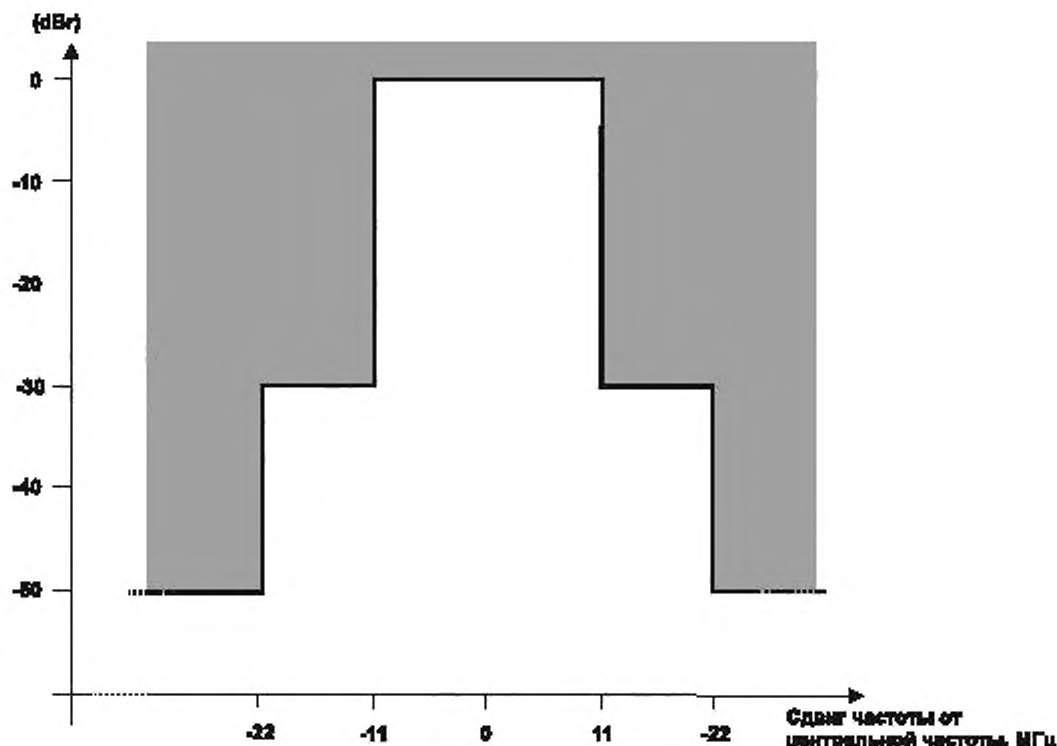
Рисунок 13 – Диапазон передаваемой СПМ в случае DQPSK-CSS
