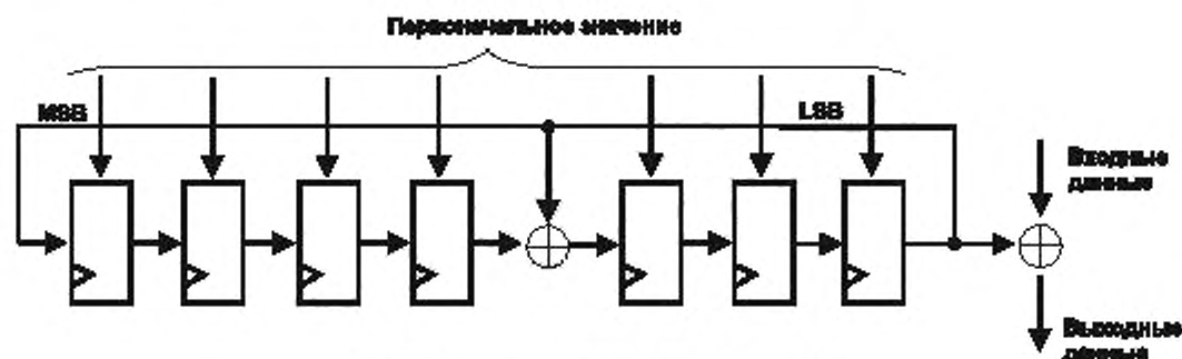
Рисунок 7 – Битовый скремблер (Bit scrambler)
