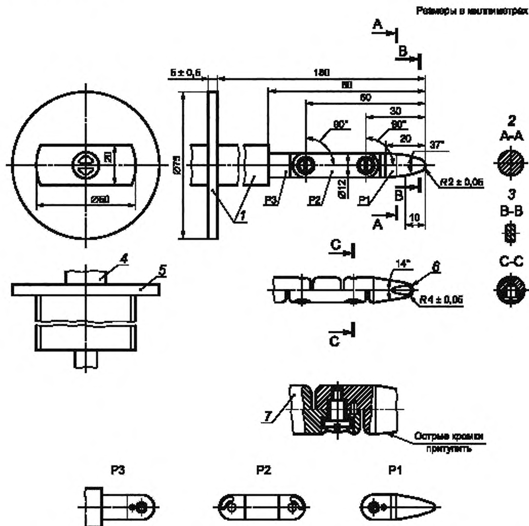
Рисунок В.2 — Шарнирный испытательный палец
