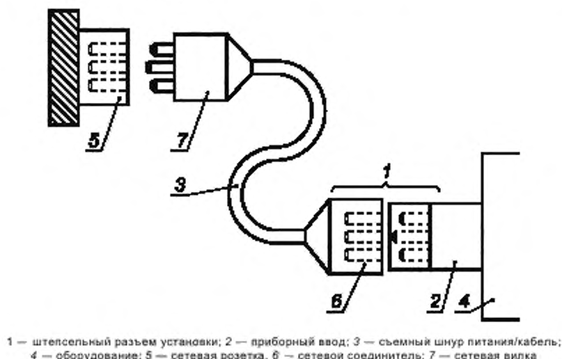
Рисунок 9 — Съемные шнуры сетевого питания и соединители
