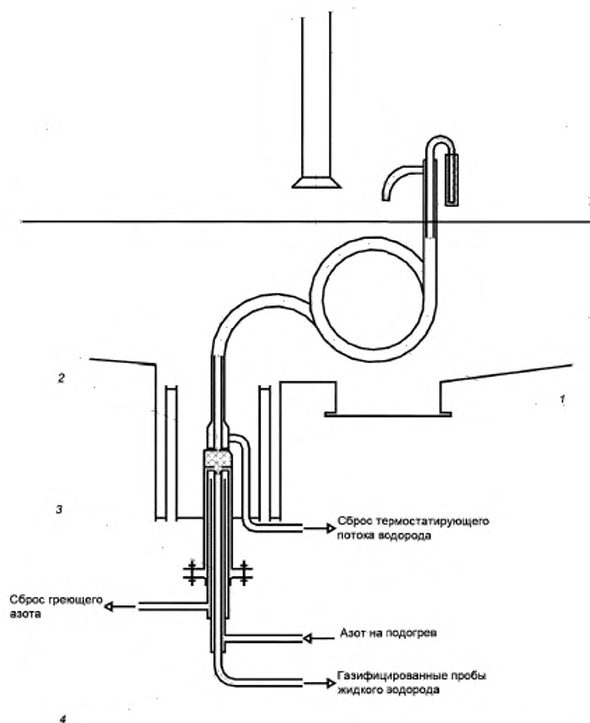
1 — термостатируемый пробоотборный трубопровод; 2 — капилляр (трубка 1х0,25 12-18Н10Т ГОСТ 14162); 3 — испаритель; 4 — анализная трубка
