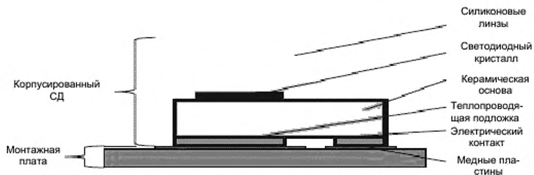
б) Поверхностный монтаж корпусированного СД без выводов
