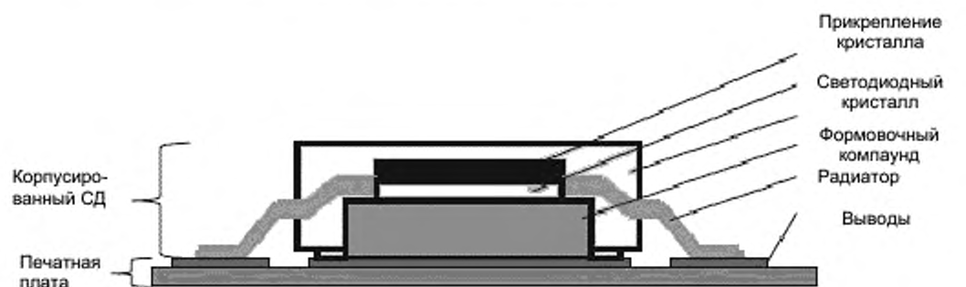
а) Поверхностный монтаж корпусированного СД с выводами
