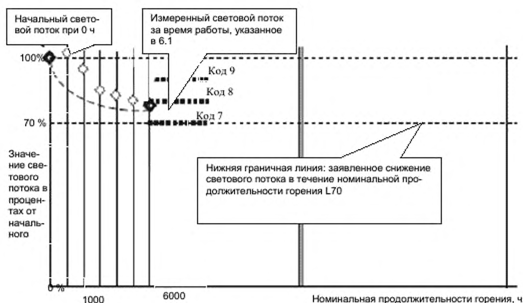
Рисунок 2 – Снижение светового потока в течение времени испытания
