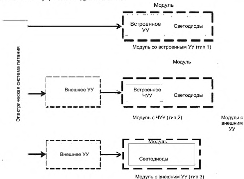
Рисунок 1 – Типы светодиодных модулей
