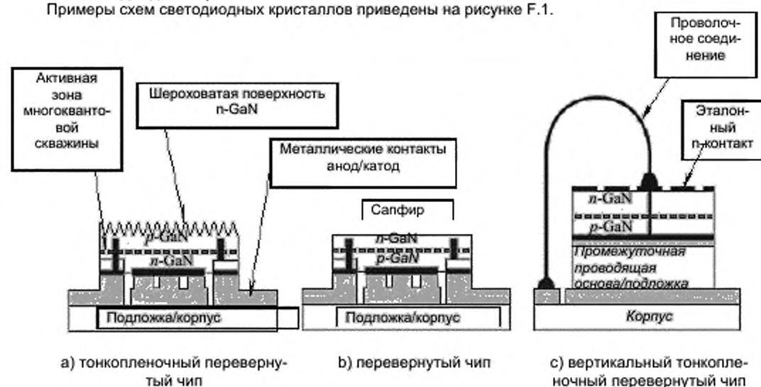
Рисунок F.1 – Схемы светодиодных кристаллов
