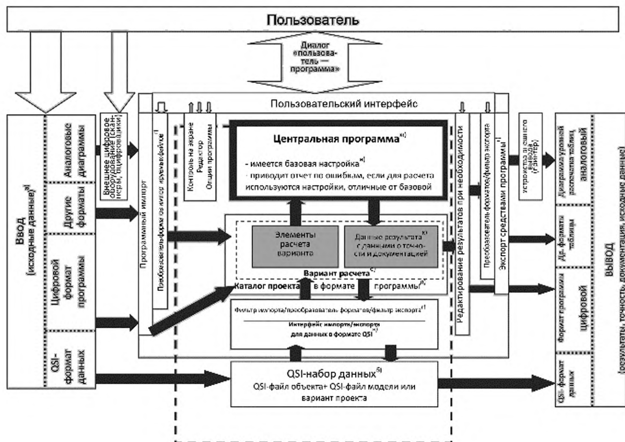
Рисунок Д.1 — Блок-схема потока данных
