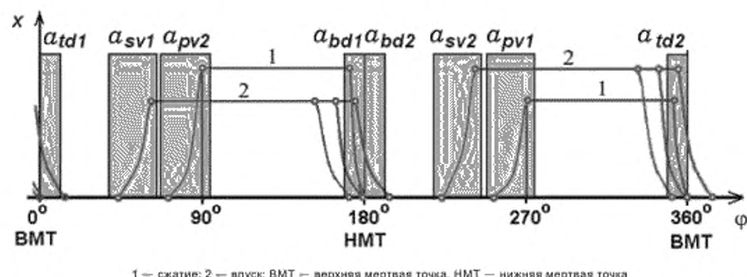
Рисунок 1 — Циклограмма работы поршневого компрессора (зависимость высоты поднятия пластины клапана от угла поворота вала)
