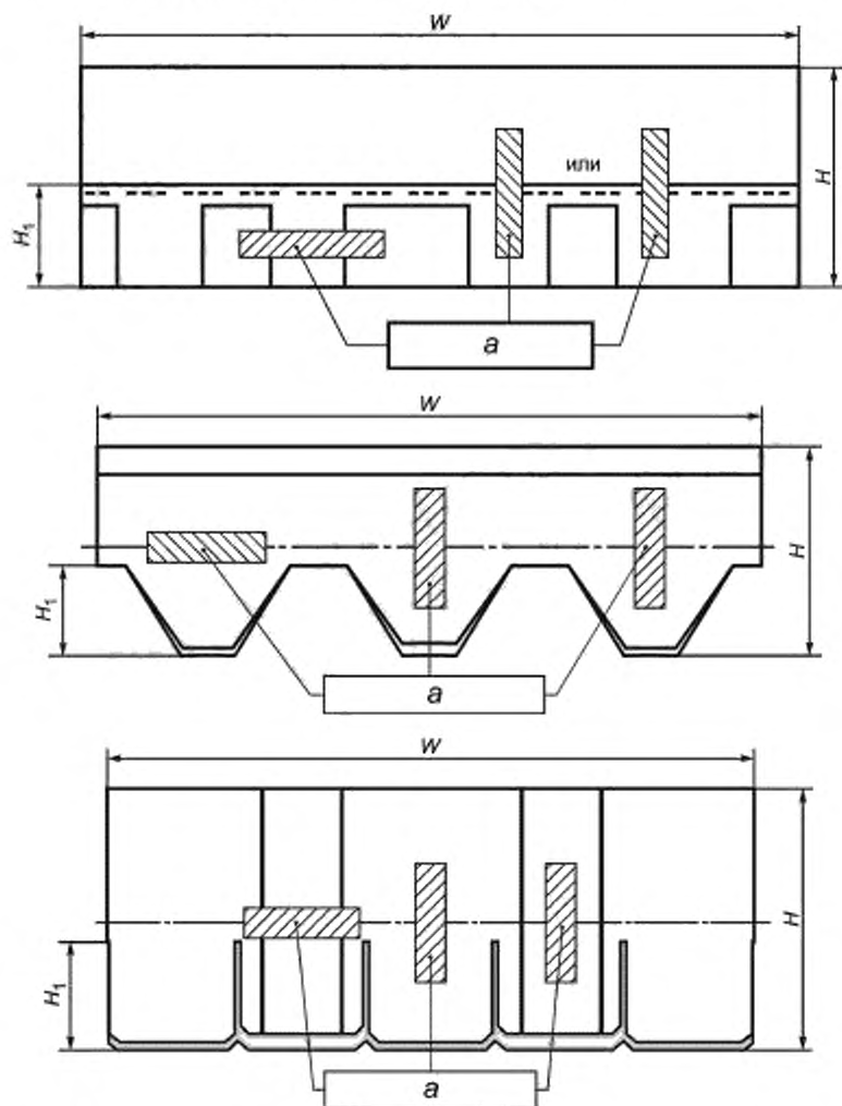
Рисунок 10 — Схема отбора образцов для двухслойной и трехслойной черепицы.
