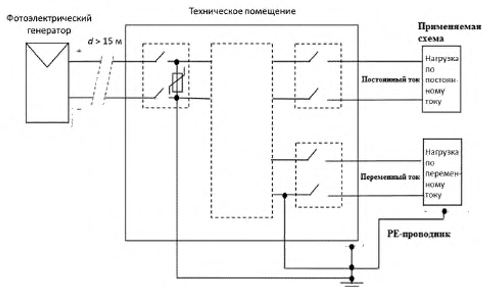
Рисунок 5 — Конфигурация Н — только солнечная фотоэлектрическая батарея индивидуальной системы электроснабжения P < 500 Вт — с инвертором — d > 15 м
