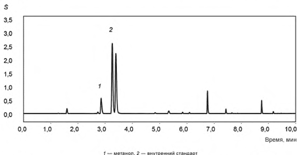
Рисунок В.2 — Хроматограмма осветленного яблочного сока прямого отжима, содержащего 160 млн -1 метанола, с добавлением 0,01 % по массе внутреннего стандарта
