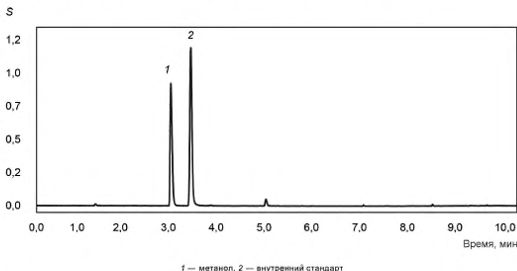
Рисунок В.1 — Хроматограмма градуировочного раствора, содержащего 250 млн -1 метанола с добавлением 0,01 % по массе внутреннего стандарта
