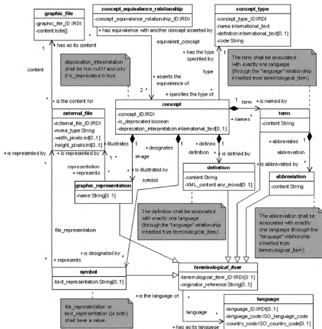
Рисунок 4 — Диаграмма класса UML для терминологии
