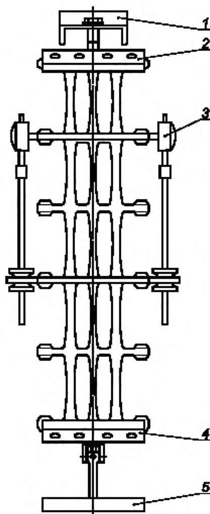
1 — жесткая рамка; 2 — верхний зажим; 3 — регулятор направления; 4 — нижний зажим; 5 — грузы
