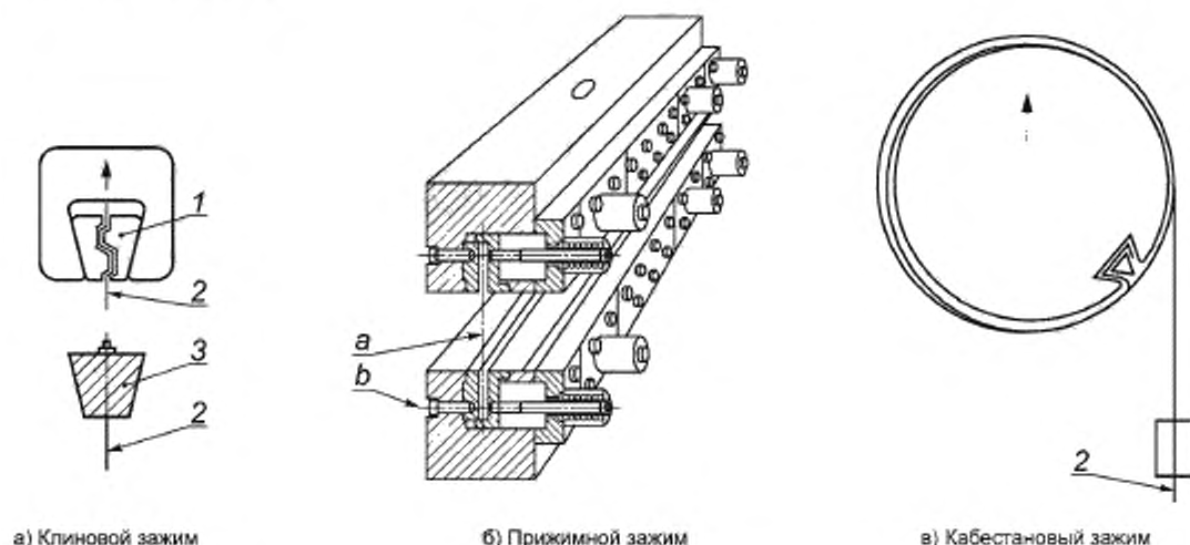
1 — зубчатый клин, 2 — геосинтетический материал; 3 — клин из эпоксидного материала или мягкого металла; а — максимальная ширина измеряемого образца 0,5 м; б — усилие зажима регулируется до 400 кН
