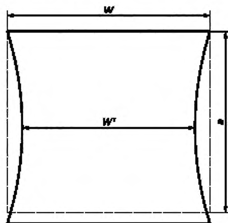
Рисунок К.2 — Размер сжатия образца
