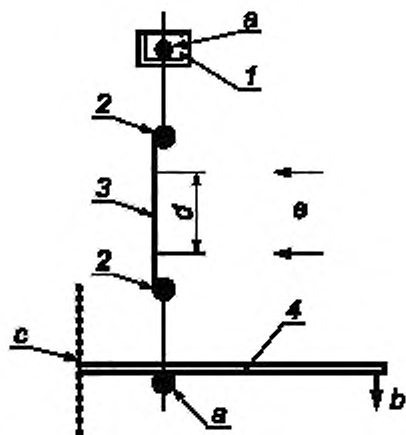
1 — жесткая рама; 2 — зажим для испытуемого образца; 3 — испытуемый образец; 4 — грузоподъемник; а — сферическая насадка; б — нагрузка; с — регулируемый центр вращения для постоянной нагрузки; d — номинальная длина; e — удаленное измерение с помощью экстензометра
