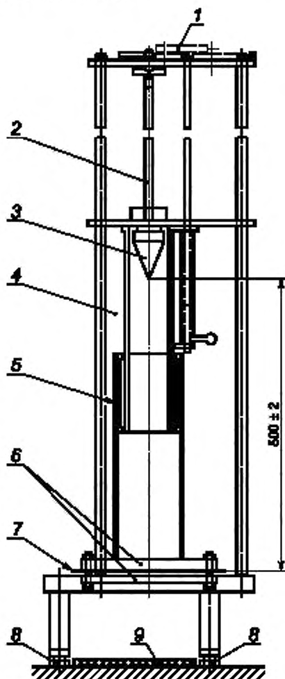
1 — верхняя часть/спусковой механизм в соответствии с требованиями лаборатории; 2 — направляющая штанга; 3 — конус; 4 — металлическая ширма; 5 — ширма; 6 — зажимные пластины; 7 — проба; 8 — регулировочный винт; 9 — защитный слой для конуса
