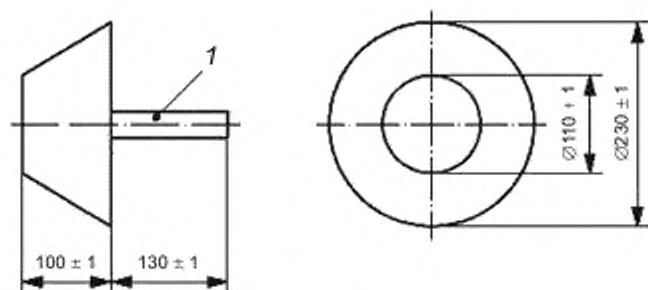
Рисунок 7 — Конусообразный щуп
