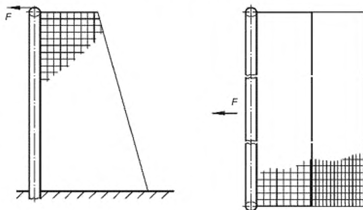
Рисунок 3 — Проверка стабильности ворот для футбола
