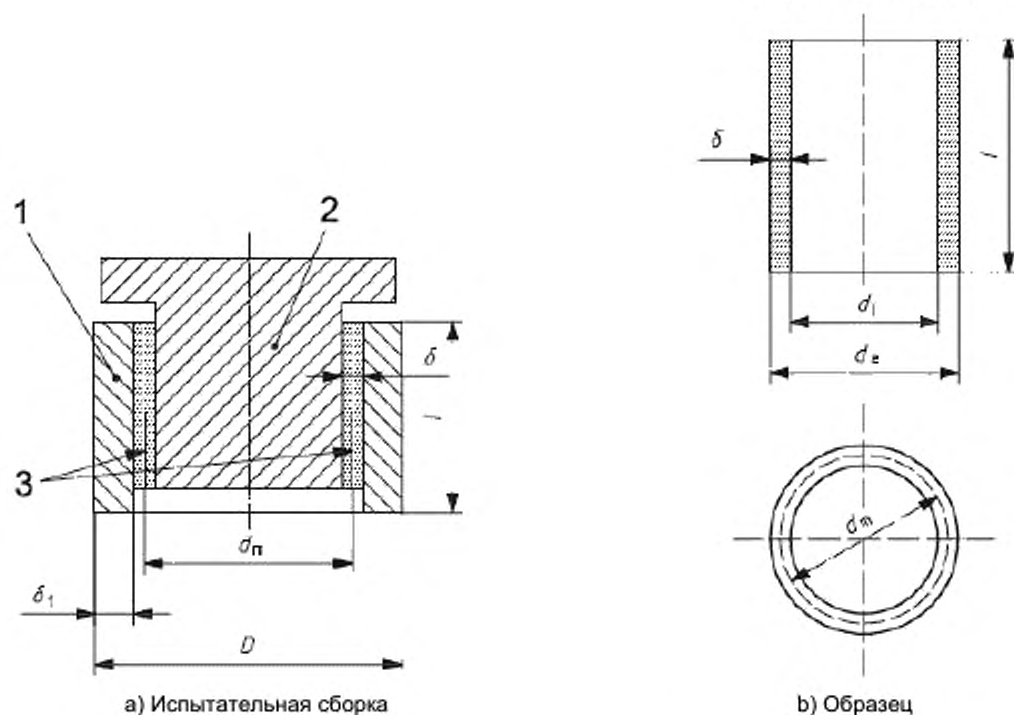
1 – поддерживающий цилиндр; 2 – поршень; 3 – образец;
