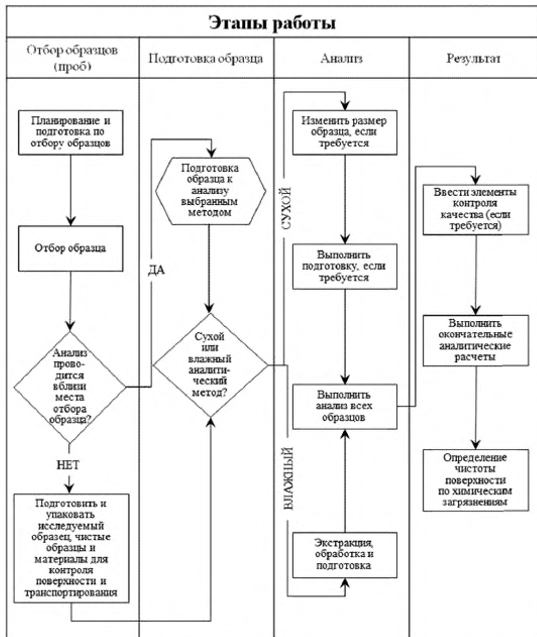
Рисунок D.3 — Схема отбора образцов (проб), анализа и контроля качества
