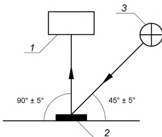
1 — спектрофотометр или колориметр для измерения координат цветности, спектрофотометр, колориметр или яркомер для измерения коэффициента яркости; 2 — ЦПП; 3 — источник света
